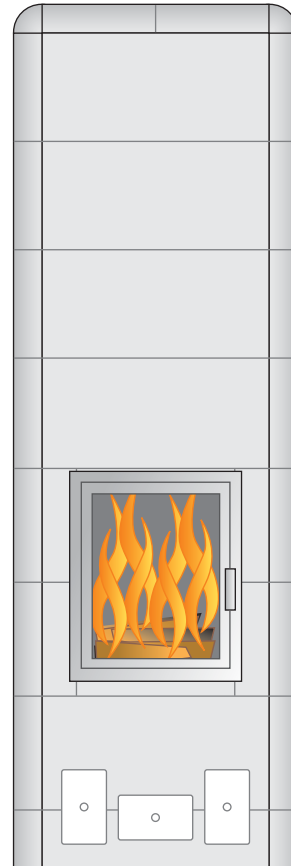
Lisävarusteena: 5 x korotus 100 mm (korkeus 2300 mm)
