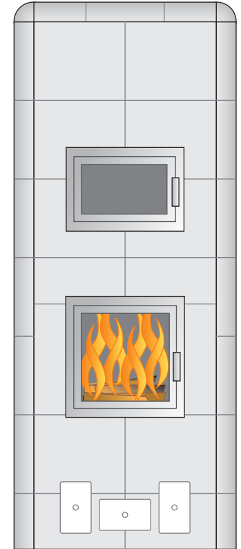
Lisävarusteena: leivinuuni 4 x korotus 100 mm (korkeus 2100 mm)
